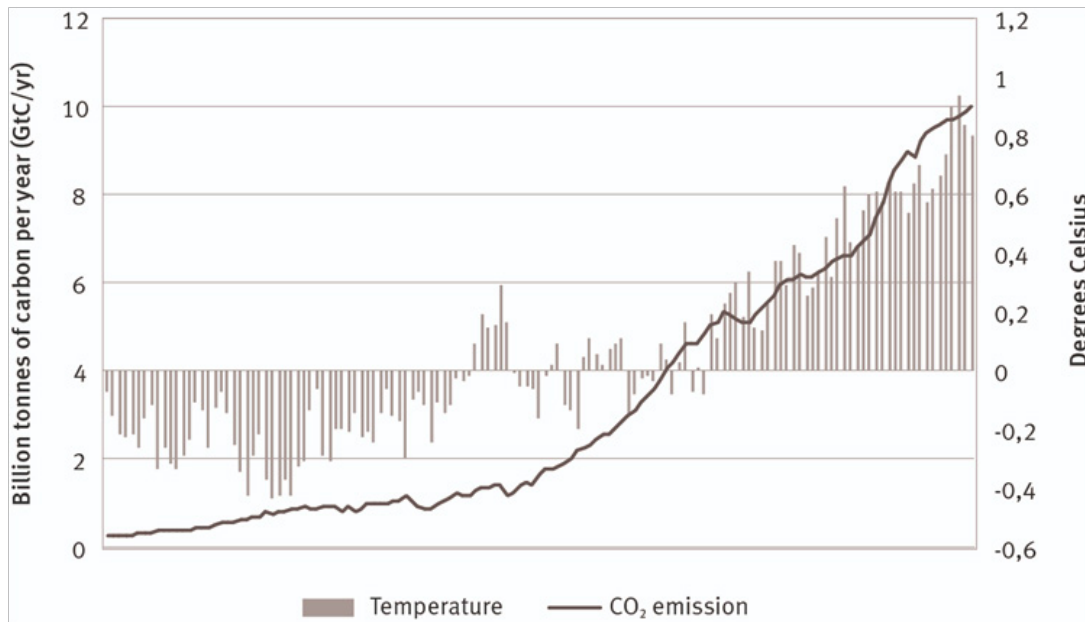
Global warming and CO 2 emissions - 1880-2015 (Aquecimento global e emissão de CO 2 - 1880-2015).
