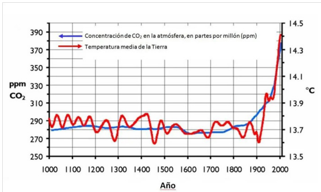
Evolución de la concentración de CO 2 atmosférico y de la temperatura media en la Tierra desde el año 1000 al 2000 (Evolução da concentração de CO 2 atmosférico e da temperatura média na Terra do ano 1000 ao ano 2000).
